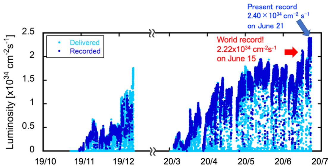
Fig. Luminosità istantanea fornita dall' acceleratore SuperKEKB al rivelatore Belle II in funzione del tempo.
